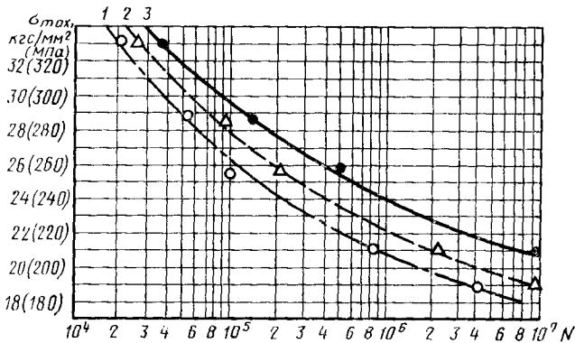
Кривые усталости образцов из сплава марки В95
